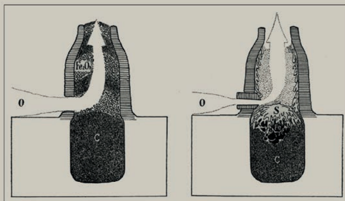
Obr. 6. Schéma redukce v latécké peci se zahloubenou nížeji. Podbořany, 1. stol. př. n. l. Vlevo počátek redukce, vpravo – konec tavby. Fe 2 O 3 – železná ruda, C – dřevěné uhlí, S – struska, O – proud vhdněného vzduchu (Pleiner 1958, 127)
